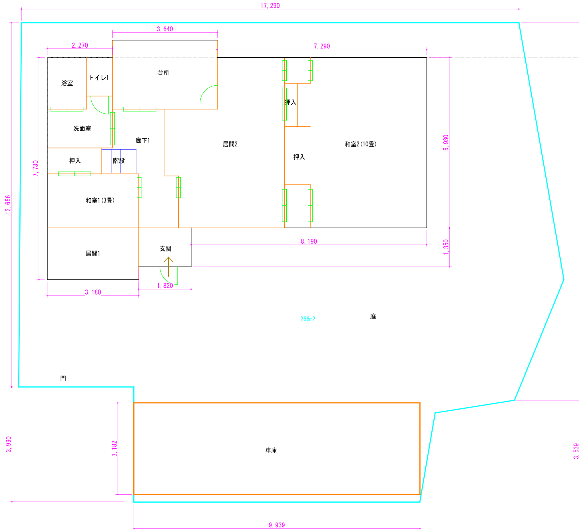
1F平面図
